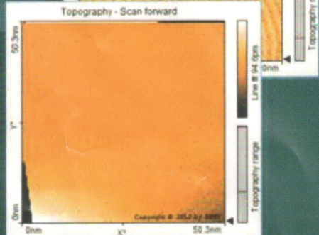
AU NANOPARTICLES
